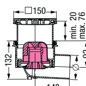
Illustrazione mostra Cod. art. 45 110.40 (scarico laterale)
